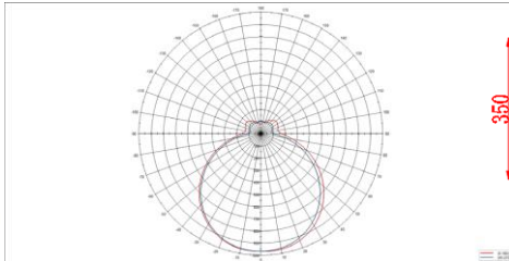
[ 배광곡선 ]
