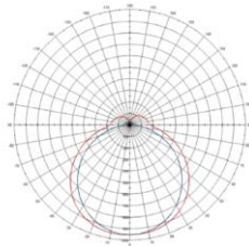
[ 배광곡선 ]
