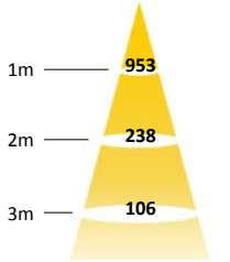
[ 조도기준 (lx) ]
